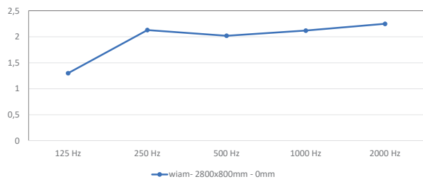
äquivalente Absorptionsfläche, m 2
